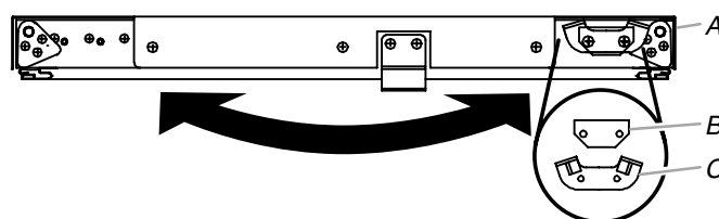
A. Parte inferior de la puerta del refrigerador B. Espaciador del retén de la puerta C. Retén de la puerta
